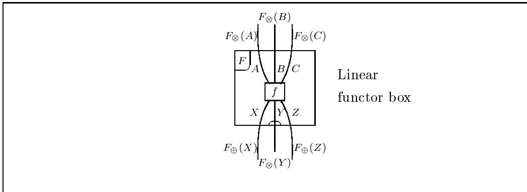
Fig. 7. Linear functor box
